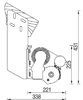
Dachsparrenbefestigung
