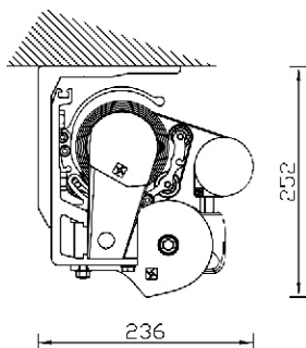
Deckenbefestigung
