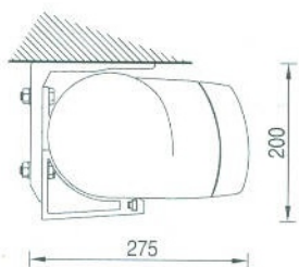
Deckenmontage
