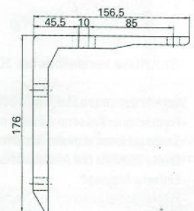
Deckenträger
