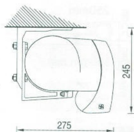
Deckenmontage mit Vario Volant
