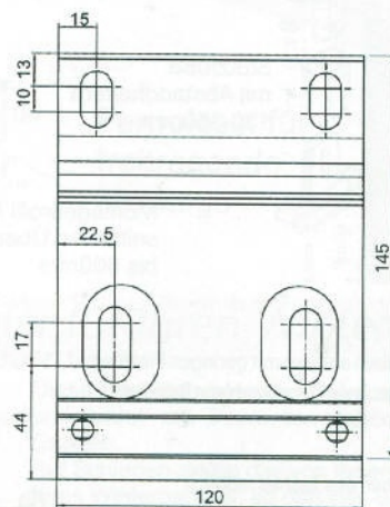
Wandträger
